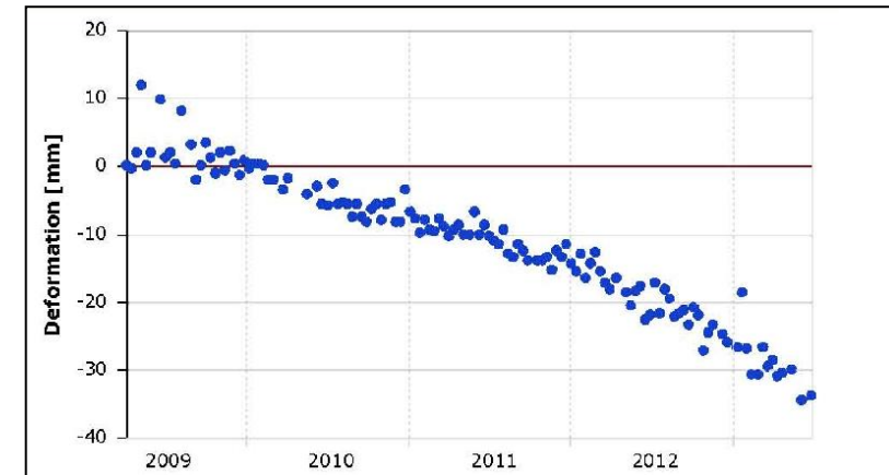
Satellietmonitoring zettingen Margrietstraat
